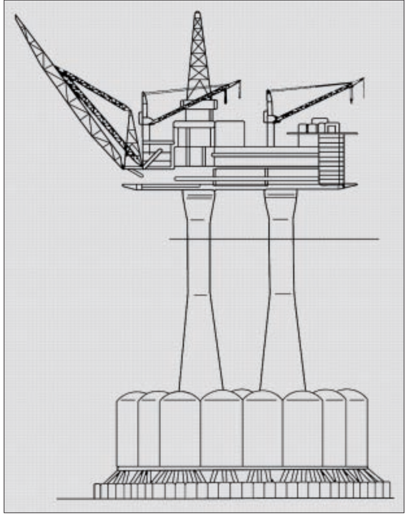
نموذج منصة «الجاكيت» التي يرتكز ظهرها على مشبك من الأنابيب والتي يعادل قطرها بضعة أمتار
